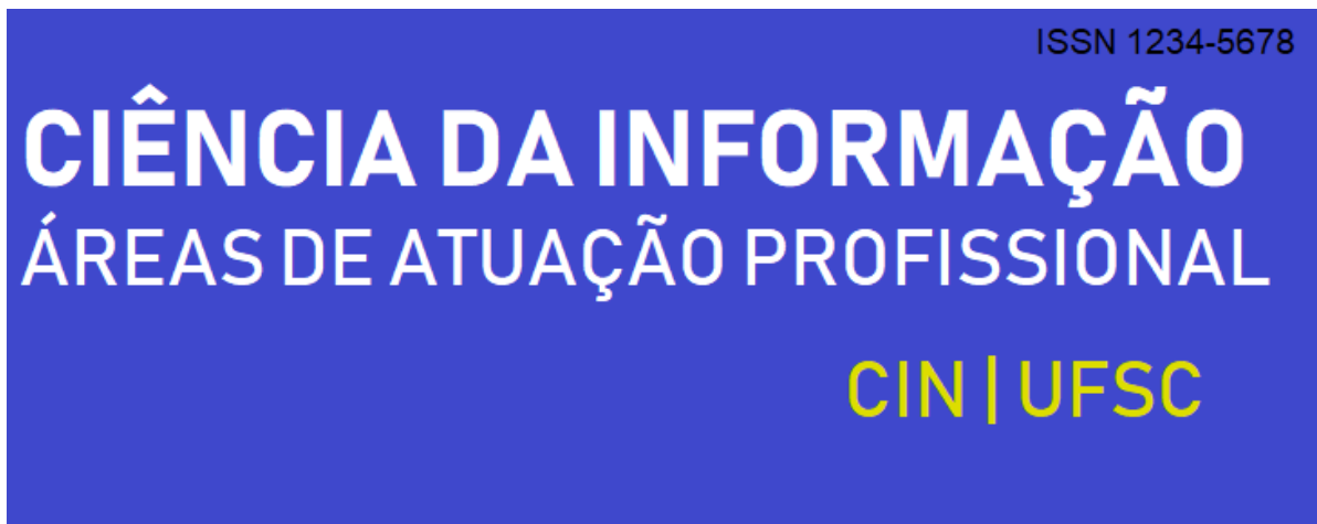
Figura 1: Cabeçalho
